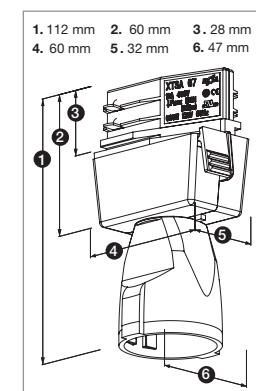
Schuko adapter 16A Adattore Schuko 16A
